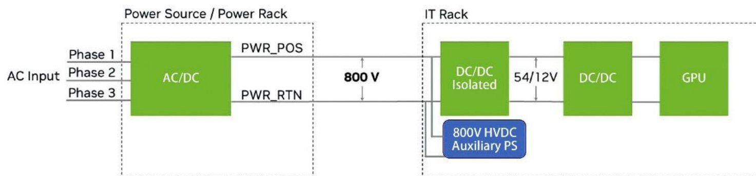
800V HVDC 輔助電源模組
